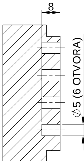
PRESEK B-B
