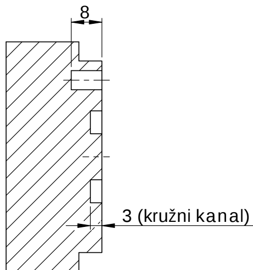
PRESEK C-C
